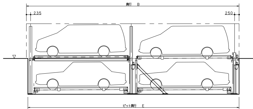
側面図
