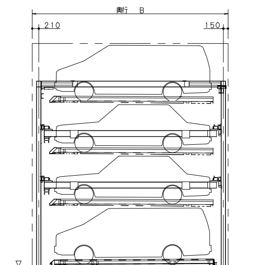
側面図
