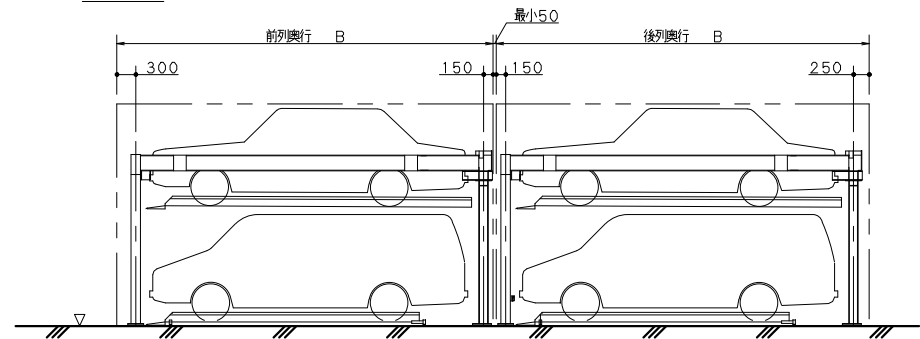
側面図
